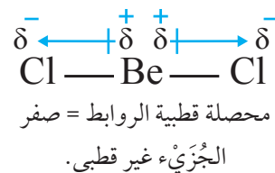
الشكل (30): العزم القطبي لجزيء BeCl_2 .
