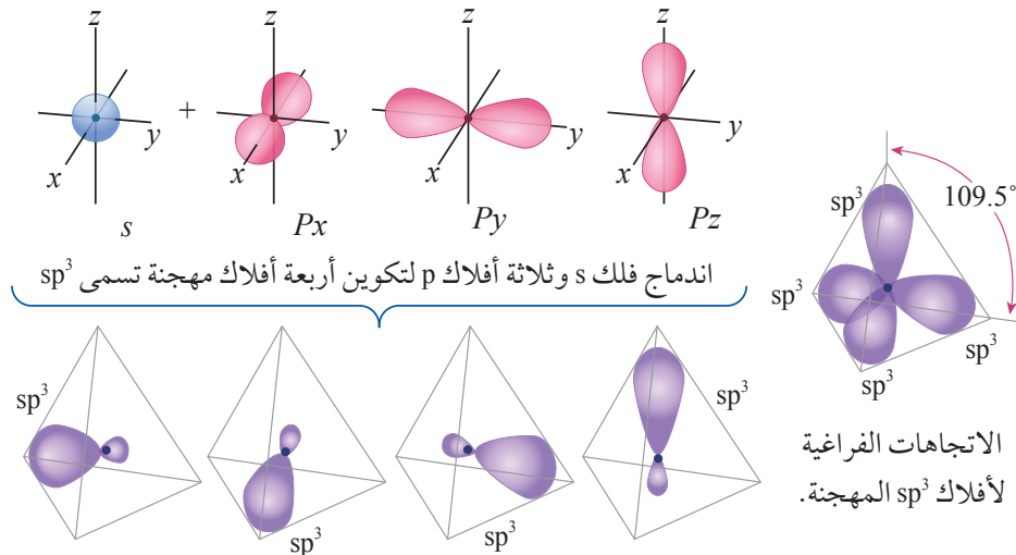
الشكل (ب/20) تكوين الأفلاك المَهَجَّنة sp^3
