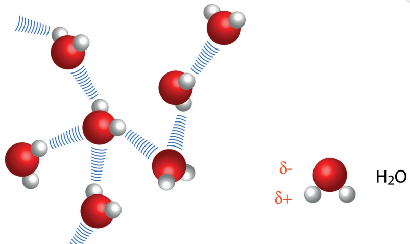
الشكل (35): الروابط الهيدروجينية بين جزيئات الماء.
