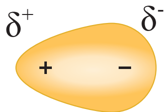
الشكل (37): الجزيء ثنائي القطب.
