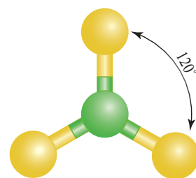
الشكل (26): الشكل الفراغي للجزيء BF_3 .
