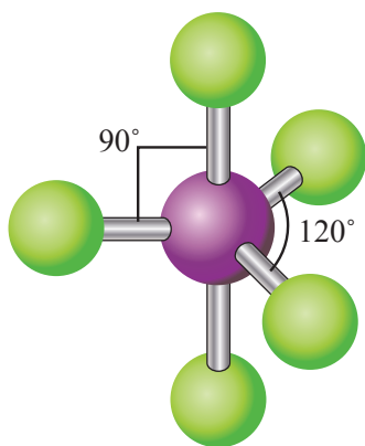
الشكل (9): تركيب لويس لجزيء \text{SF}_6 وشكله الفراغي.
