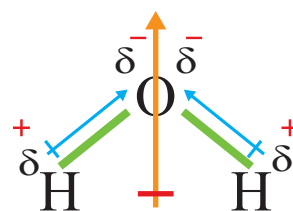
الشكل (31): العزم القطبي لجزيء H_2O .
