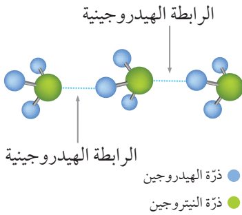
الشكل (34): الروابط الهيدروجينية بين جزيئات الأمونيا.
