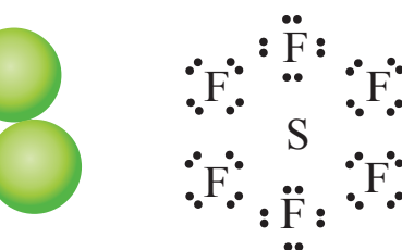
الشكل (9): تركيب لويس لجزيء \text{SF}_6 وشكله الفراغي.
