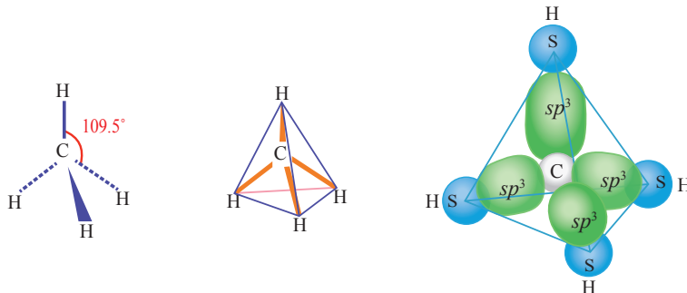
الشكل (22): الأفلاك المتداخلة لتكوين الروابط في جزيء CH_4 .
