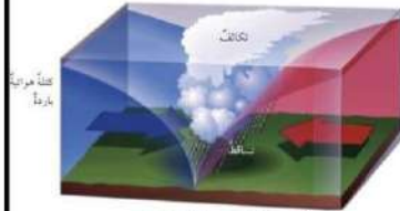
الشكل (8): تهيئة حدوث الامطار الإعصارية.
