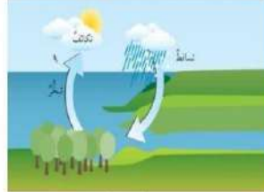
الشكل (9): تهيئة حدوث الامطار الجبلية.
