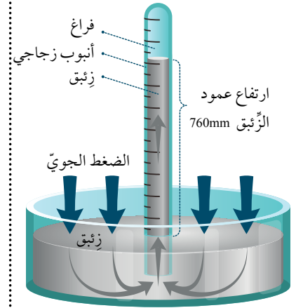
الشكل (19/أ): بارومتر توريشلي لقياس الضغط الجوي. أستخدم مبدأ عمل بارومتر توريشلي في قياس الضغط الجوي
