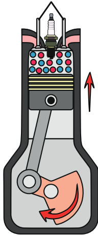
الشكل (3): شوط الضغط.
