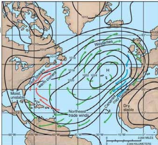
الشكل (9): مرتفع أزوري يتمركز فوق المحيط الأطلسي بالقرب من جزر الأزور البرتغالية الضغط الجوي في مركزه 1024 مليبار.
