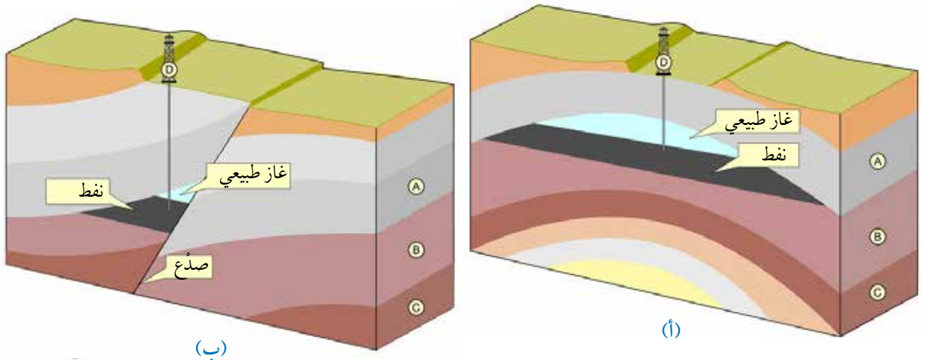
الشكل (4) تتشكل المصائد التركيبية نتيجة العمليات التكتونية التي يتعرض لها الصخر، ومن أمثلتها: أ- الطيات المحدبة ب- الصدوع
