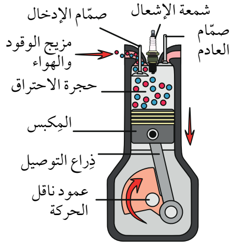
الشكل (1): أجزاء محرك الاحتراق الداخلي.
