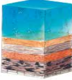
تحول المادة العضوية الى نفط أو غاز طبيعي
