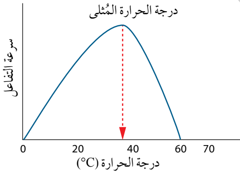
الشكل (28): أثر درجة الحرارة في سرعة تفاعل يُحفّزه إنزيم. أتتبع تأثير سرعة تفاعل يُحفّزه إنزيم بزيادة درجة الحرارة.
