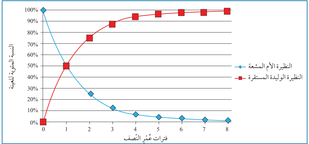
الشكل (21): تتحول النظيرة الأم المشعة عن طريق الاضمحلال الإشعاعي إلى نظيرة وليدة مستقرة. أقارن بين منحنى كل من النظيرة الأم المشعة المتبقية، والنظيرة الوليدة المستقرة في فترة عُمر النصف الثانية.
