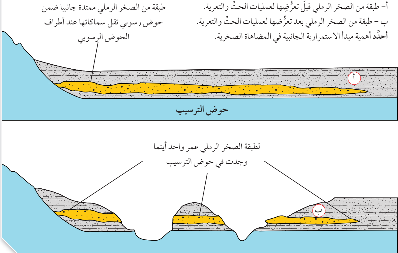
الشكل (14): مبدأ الاستمرارية الجانبية
