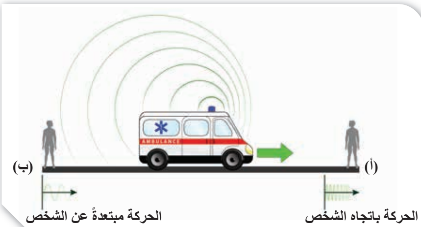
الشكل (11): تأثير دوبلر.
