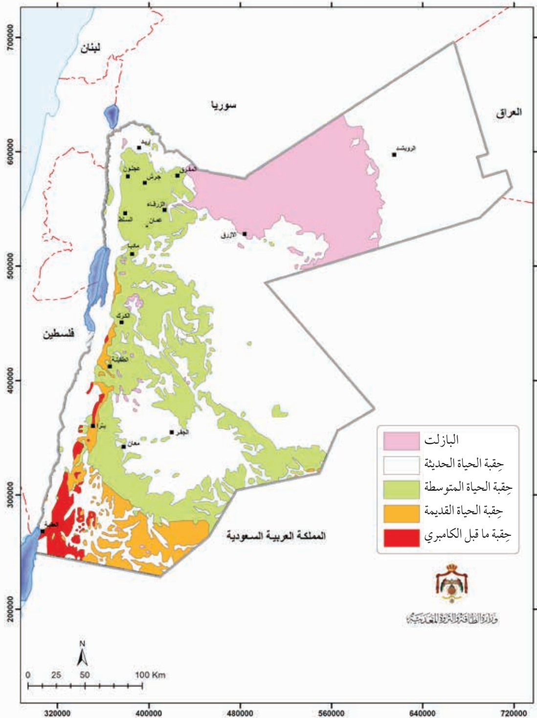
الشكل (34): خريطة الأردنّ تُظهرُ توزُّع الصخور بحسب الحِقب التي تتبع لها. أحدّد: أين تتكتشف صخور حِقبة ما قبل الكامبري في الأردنّ؟
