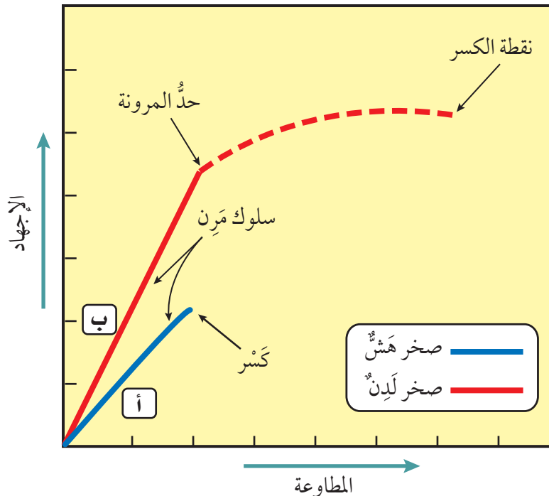
الشكل (2): الإجهاد والمطاوعة في الصّخور الهشّة واللدّنة. أبينّ ماذا يحدث للصّخور اللدّنة بعد استمرار تعرّضها للإجهاد الذي يزيد على حدّ المرونة.
